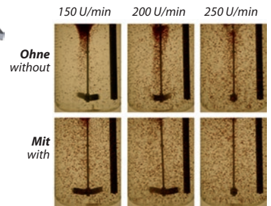
Einziehen von aufschwimmenden Feststoffen Dragdown of floating particles
